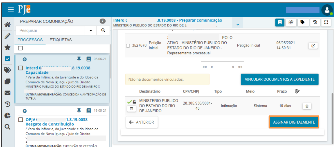
Figura 71 – Opte por um método de assinatura.
