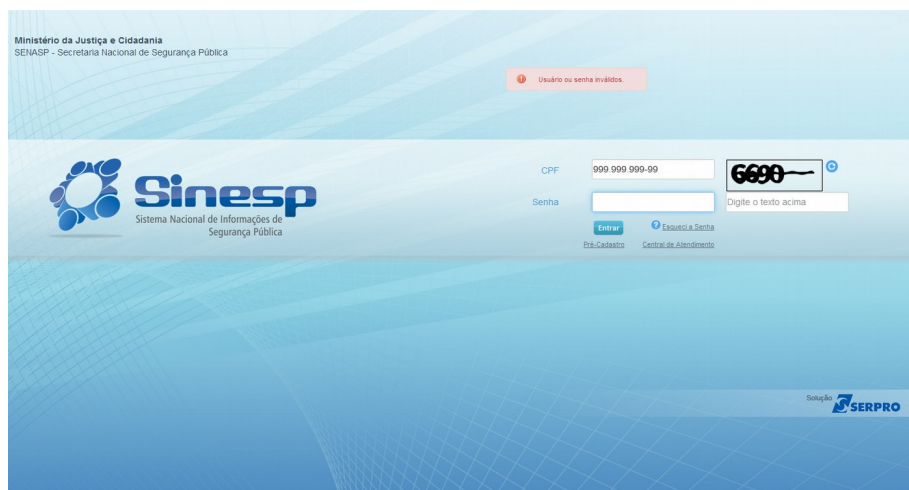
Figura 3: Senha Inválida
