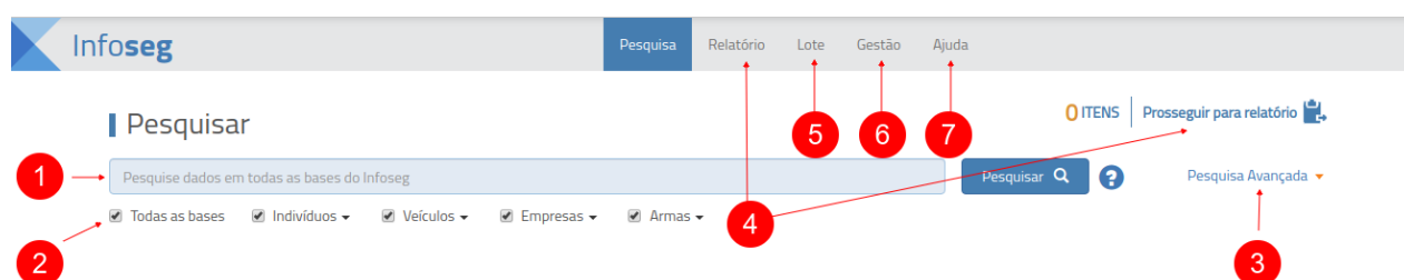
Figura 5: Tela Inicial
